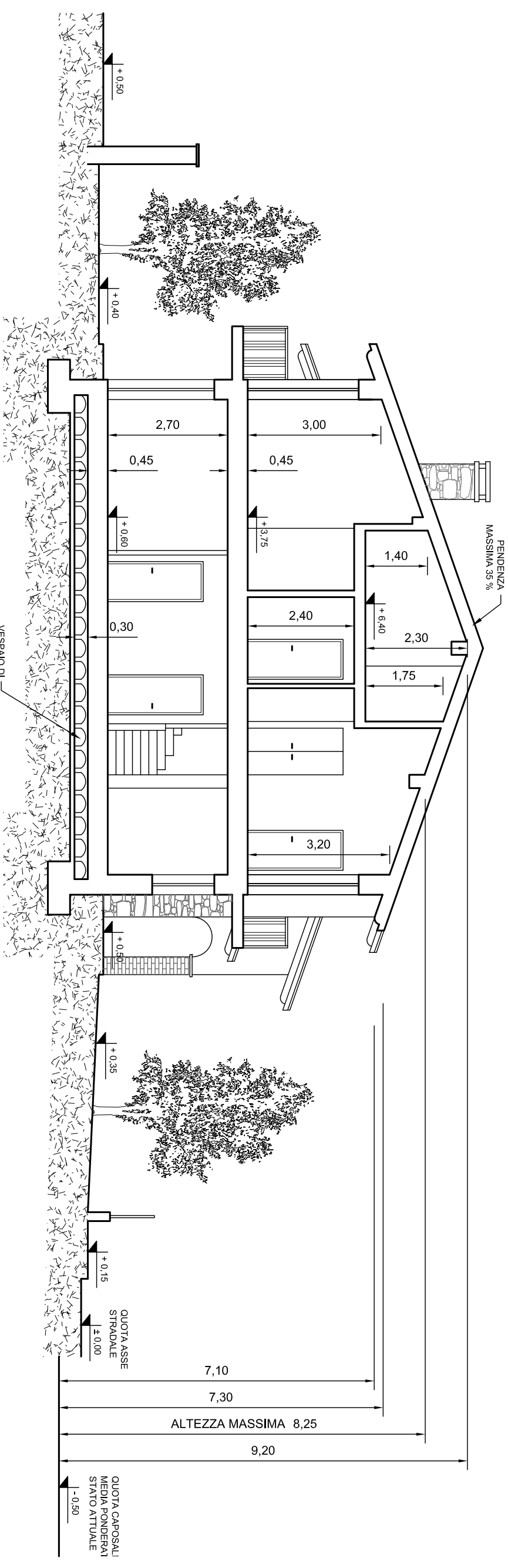
SEZIONE A - A SCALA 1:100
